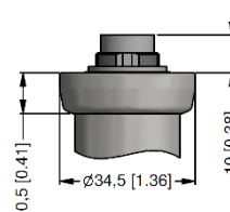
Binder Serie 723, 5-pin (IP 67)
