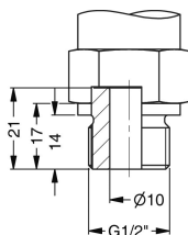
G1/2" 开放式接口 P_N \leq 40 bar
