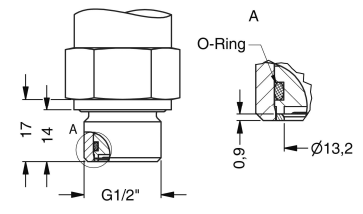
G1/2" DIN 3852 带平齐传感器 P_N \leq 40 bar
